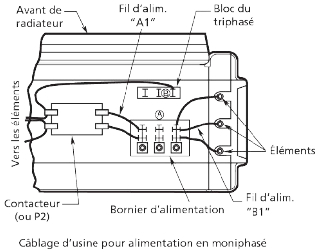
Figure 3a. Raccordements d'alimentation pour du secteur monophasé et triphasé (HUHAA520FC, HUHAA524FC, HUHAA720FC)
