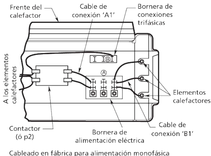
Figura 3a. Conexiones de cables para alimentación monofásica y trifásica (HUHAA520FC, HUHAA524FC, HUHAA720FC)
