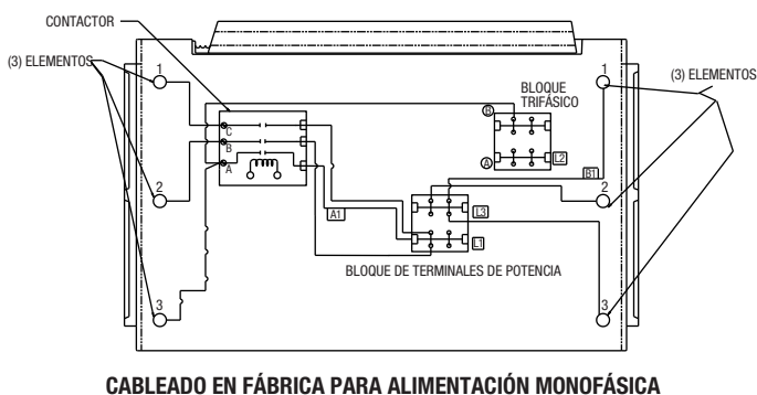
Figura 3b. Conexiones de cableado para alimentación monofásica y trifásica (HUHAA520FC, HUHAA524FC, HUHAA720FC)
